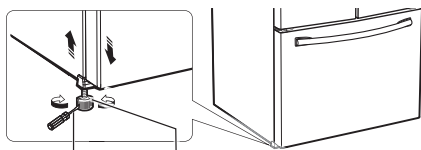
Tournevis à tête plate (-) Molette
